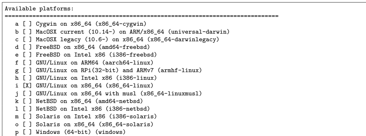
FIGURE 5 – Menu pour le choix des binaires
