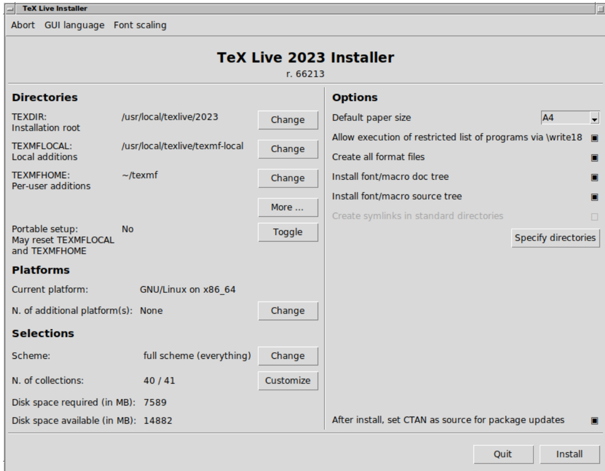
FIGURE 4 – Fenêtre de installateur en mode GUI avancé (GNU/Linux)
